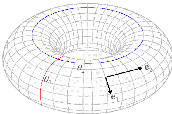
شکل ۱۰: یک چنبره و بردارهای مماس بر آن.
