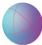
هندسه غیر اقلیدسی (بیضوی)، انحنای یکنواخت و مثبت، مجموع زوایای هر مثلث بیش از ۱۸۰ درجه است.
